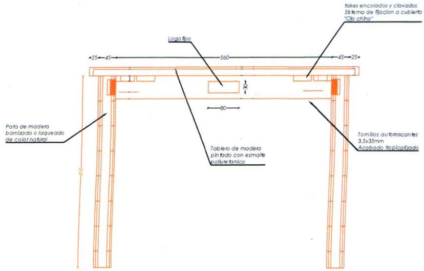
ELEVACION LATERAL
