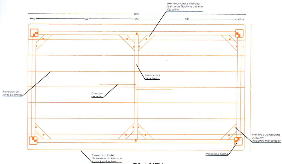
PLANTA
